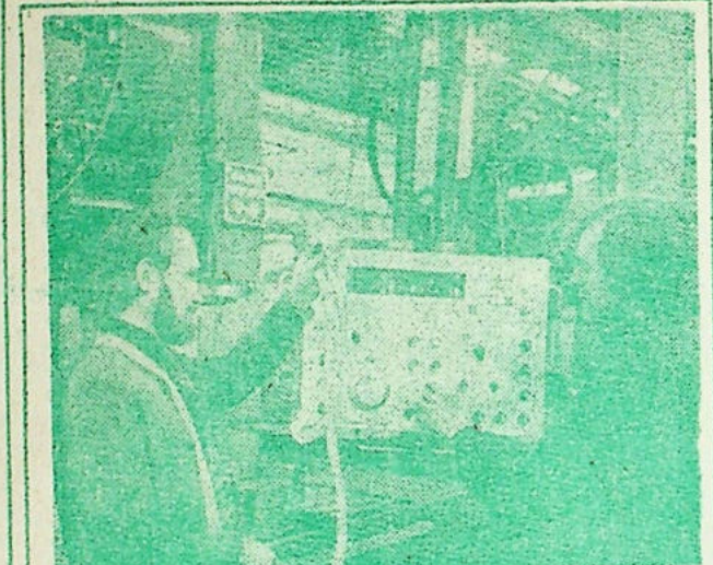
Vilniaus „Komunara“ staklių gamykloje baigtos montuoti staklės su programiniu valdymu. Įvedus specialią perforuotą, staklės pačios parenka darbo režimą. Šiomis staklėmis bus apdorojami staklių korpusai, joms galima frezuoti, grežti, lankinti.
