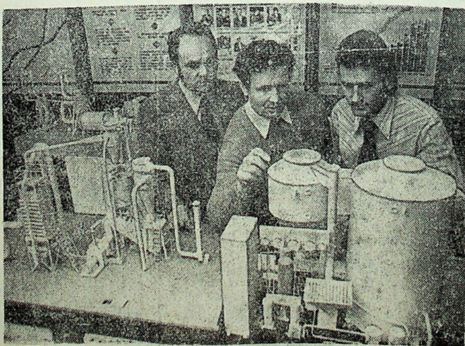
Maždaug dvigubai padidėjo šiaudų maistingumas, apdorojus juos kaustine soda. Tokią technologinę liniją sukūrė Zolės ir šiaudų perdirbimo mašinų pagrindinio eksperimentinio konstravimo instituto Vilniuje specialistai.
