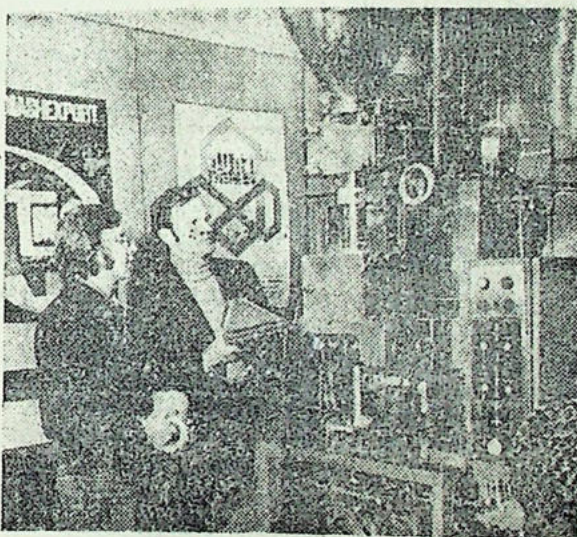
NUOTRAUKOJE: įpakavimo automato žinybinės laboratorijos (iš dešinės) vedėjas L. Paulauskas ir jaunesnysis mokslinis bendradarbis R. Danilevičius bando šioje laboratorijoje sukonstruotą automatą, kuris įsuičia dešras į sintetinę plėvelę.
