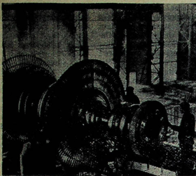
KINIJOS LIAUDIES RESPUBLIKA. Charbino turbogeneratorių gamykloje pagaminta pirmoji šalyje 100 tūkstančių kilovatų galingumo garo turbina. Nuotraukoje: statomas turbinos rotorius.
