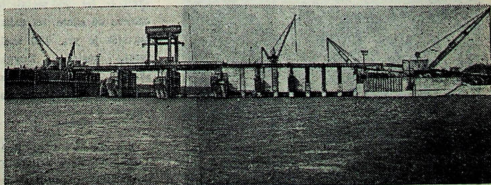
Nuotraukoje: Kauno jūra prie HES slenkstinės užtvankos. M. Ogajaus (ELTOS) nuotr.
